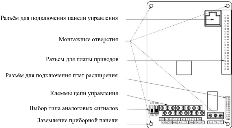
Рис. 3-20 Плат управления (стандартная)
