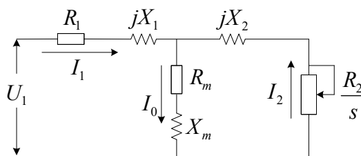
Рис. 6-12 Эквивалентная схема асинхронного двигателя
