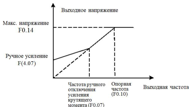
Рис.6-10 Схема усиления крутящего момента
