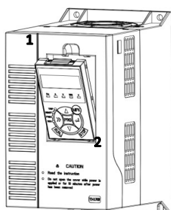
Рис.2-4 Снятие клавиатуры
