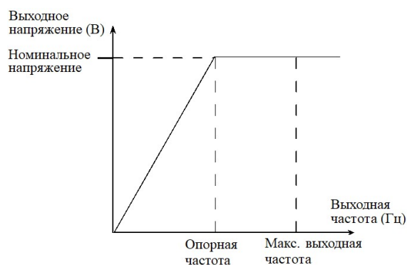
Рис. 6-1 Диаграмма зависимости V/F (вольт-частотная характеристика)
