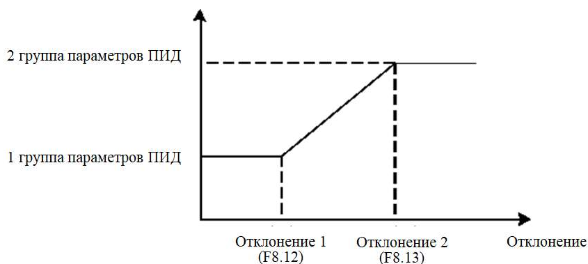
Рис. 6-24 Переключение параметров ПИД
