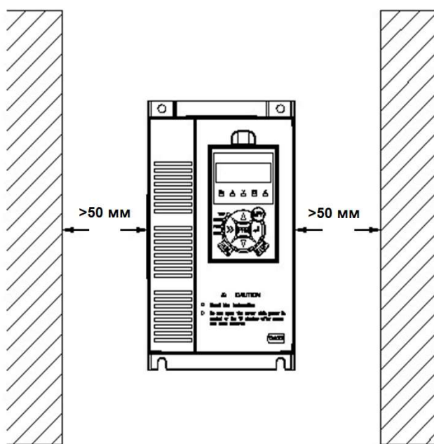
Рис.2-1 Положение при установке
