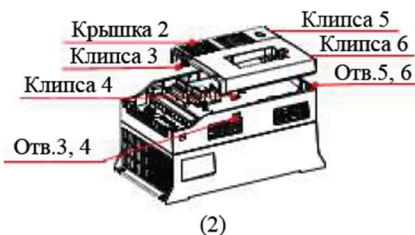
Рис.2-8 (б) ITD...B3 (15~22 кВт)
