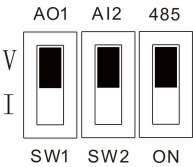
Рис. 3-22 Настройка двухпозиционного переключателя
