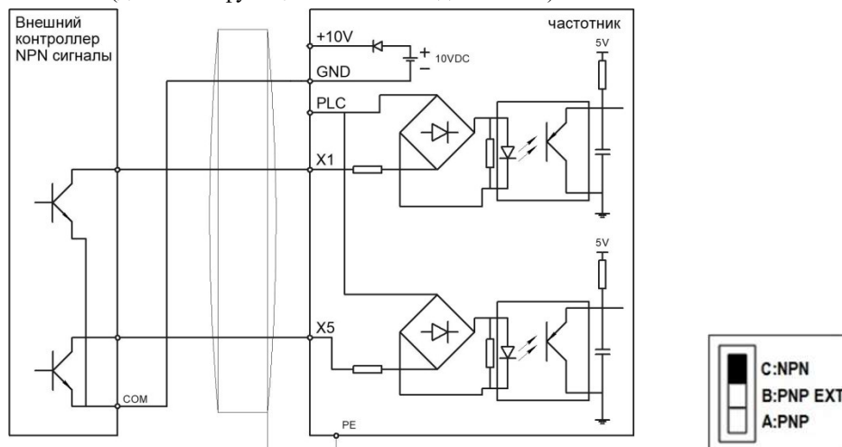
Рис. 3-13 Стандартный способ подключения NPN с помощью проводов эмиттера
