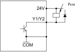
Рис. 3-16 Способ подключения внутреннего источника питания +24 В
