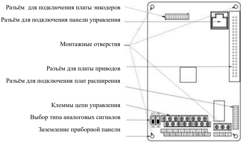
Рис. 3-21 Плата управления с возможностью подключения платы энкодеров
