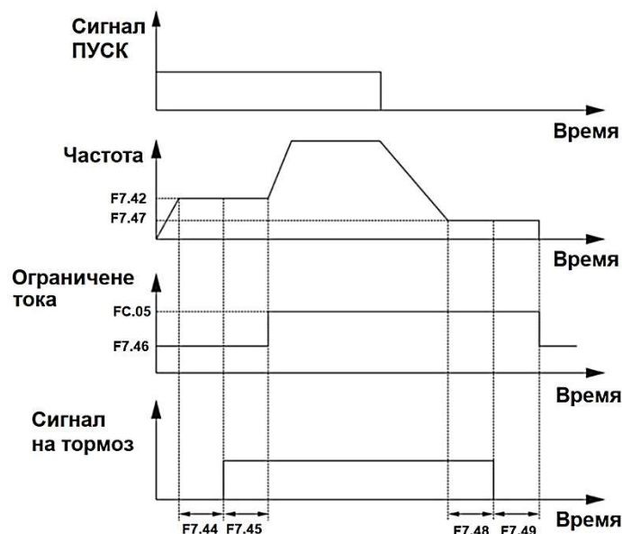
Рис. 6-23 Сигнал управления двигателем с электромеханическим тормозом
