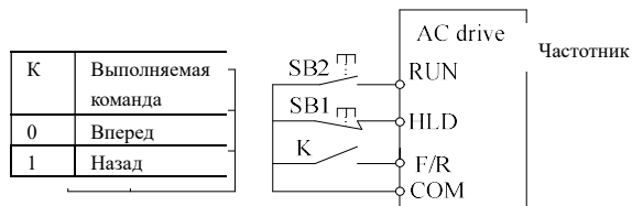
Рис.6-16 Трехпроводной режим управления 2
