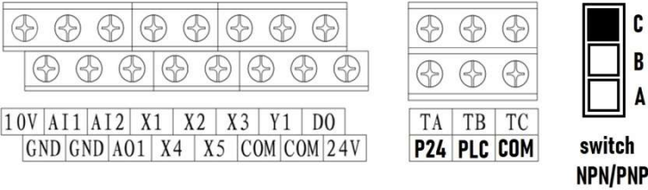
Рис. 3-10 Расположение клемм цепи управления для версии B2_0102/0302
