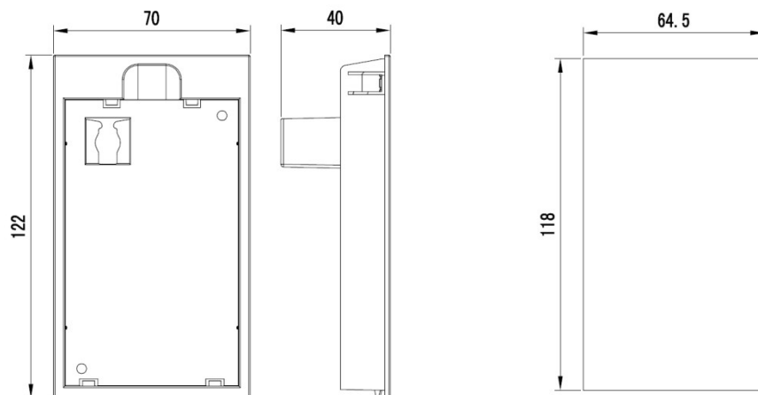
Рис.1-4 Чертеж полки для пульта управления и монтажные размеры
