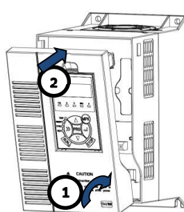
Рис.2-7 Установка пластикового корпуса
