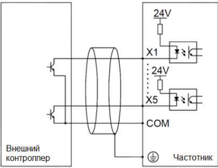
Рис. 3-12 Стандартный способ подключения NPN с помощью проводов эмиттера
