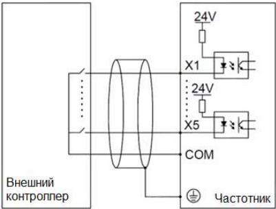
Рис. 3-11 Схема подключения цепи управления
