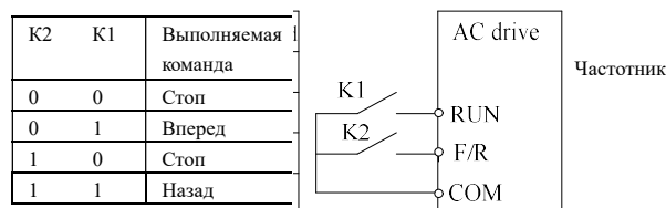
Рис. 6-14 Двухпроводной режим управления 2
