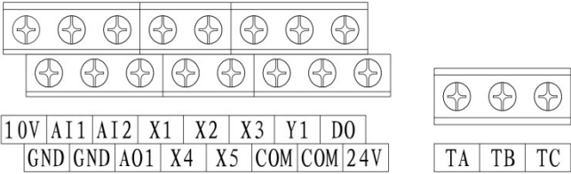
Рис. 3-9 Расположение клемм цепи управления
