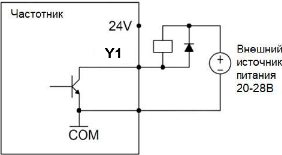
Рис.3-17 Способ подключения внешнего источника питания
