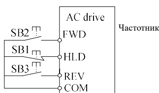
Рис.6-15 Трехпроводной режим управления 1
