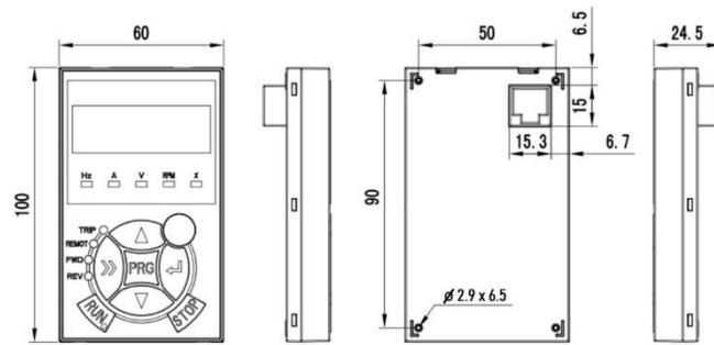
Рис.1-3 Схема пульта управления и монтажные размеры
