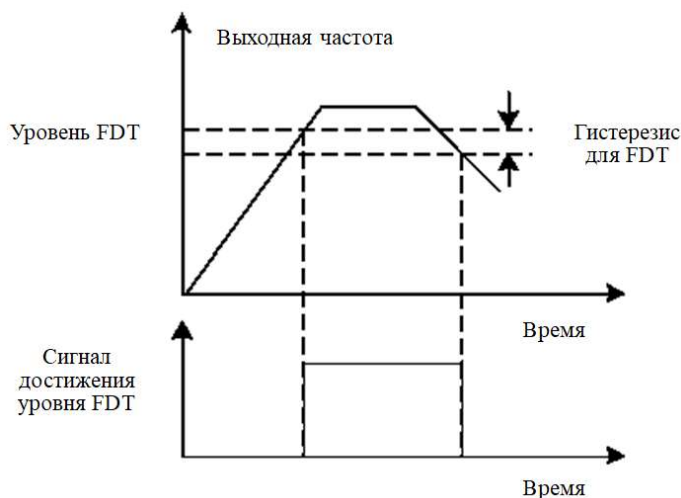
Рис. 6-21 Уровень FDT и схема задержки
