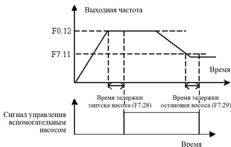
Рис. 6-22 Сигнал управления вспомогательным насосом для постоянной подачи воды под давлением
