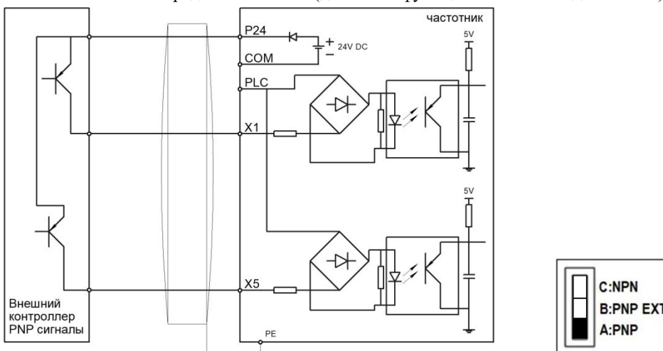
Рис. 3-15 Стандартный способ подключения PNP с внутренним источником питания 24VDC
