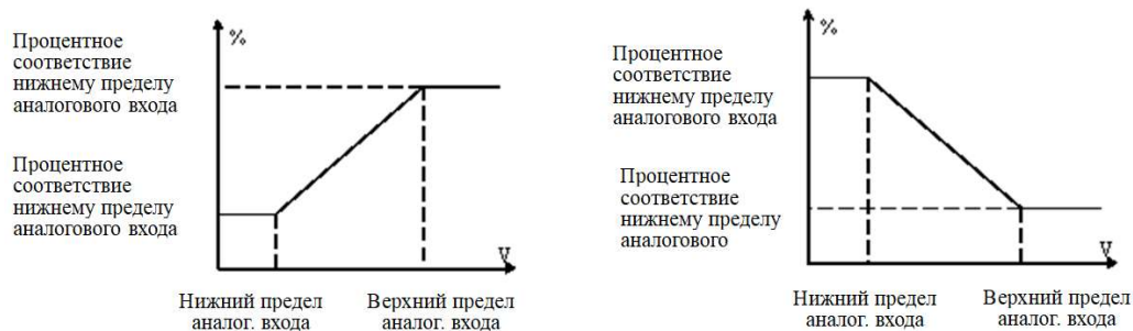
Рис. 6-18 Линейная кривая аналогового входа
