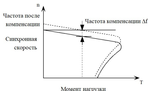
Рис. 6-11 Автоматическая компенсация скольжения
