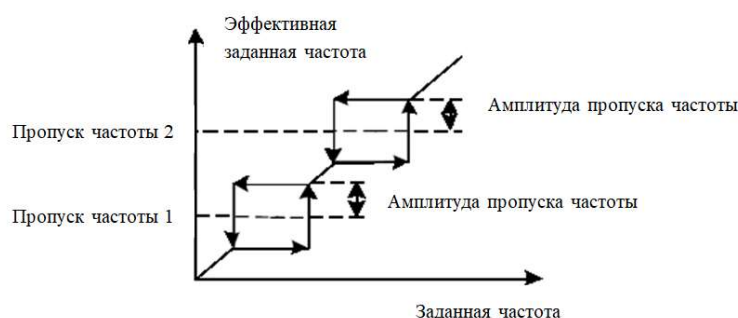
Рис. 6-5 Пропуск частот
