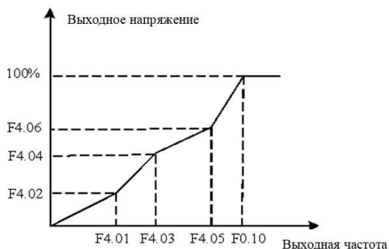
Рис.6-9 Кривая зависимости напряжения от частоты, определяемая пользователем
