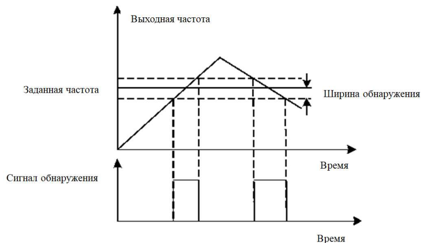
Рис.6-20 Схема обнаружения FAR
