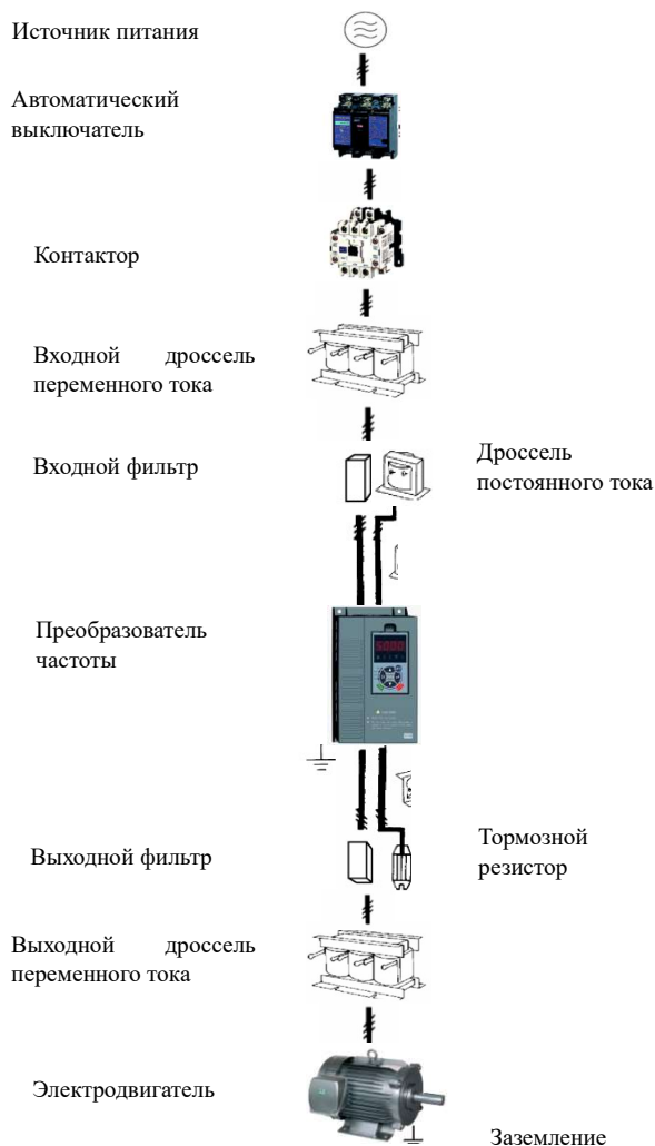
Рис 3-1 Подключение периферийных устройств к преобразователю
