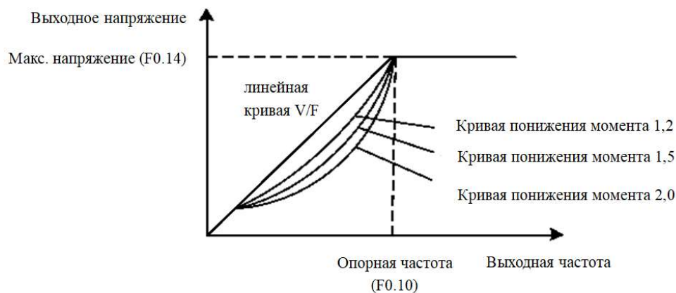
Рис. 6-8 Кривая понижения крутящего момента
