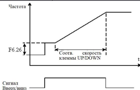
Рис. 6-19 Начальный шаг клеммы UP/DOWN
