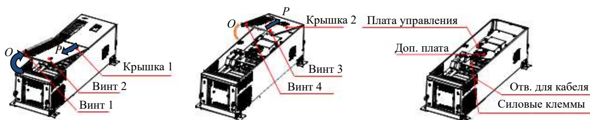
Рис.2-10 ITD...B3 (160~315 кВт)
