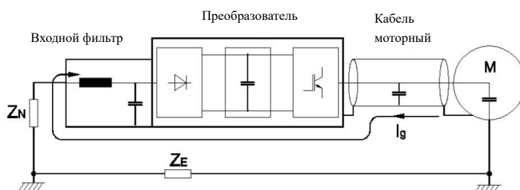
Рис. 3-6 Меры по борьбе с помехами
