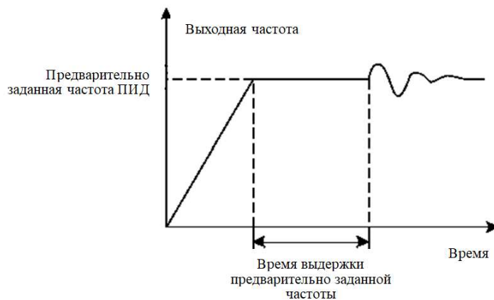
Рис. 6-25 Предварительно заданная частота и время выдержки предварительно заданной частоты ПИД
