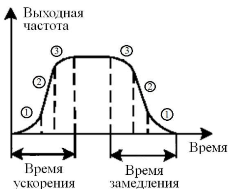
Рис. 6-4 Ускорения/замедление на S-кривой
