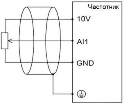
Рис. 3-18 Подключение аналоговых входов
