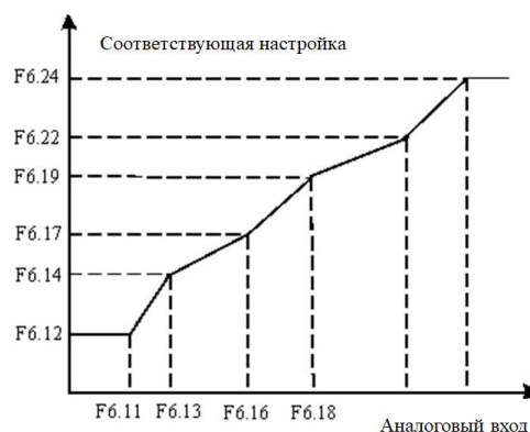
Рис. 6-17 Нелинейная кривая аналогового входа
