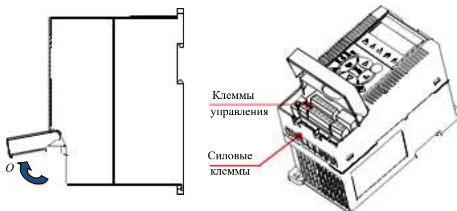
Рис.2-3 ITD...B2 (0.25~1.5 кВт)
