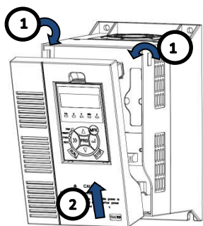
Рис.2-6 Снятие пластикового корпуса
