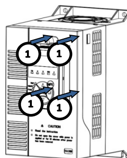
Рис.2-5 Установка клавиатуры
