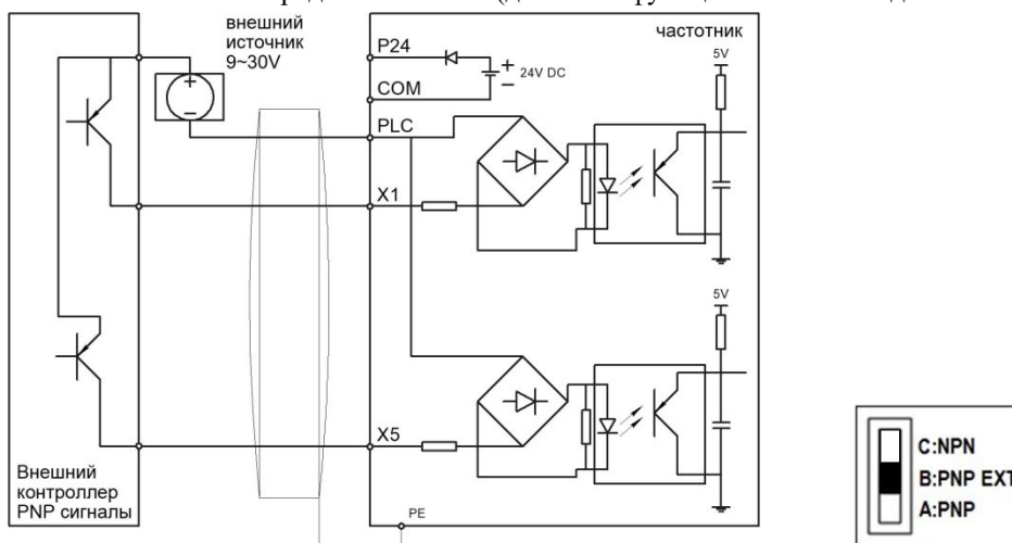
Рис. 3-14 Стандартный способ подключения PNP с внешним источником питания 24VDC
