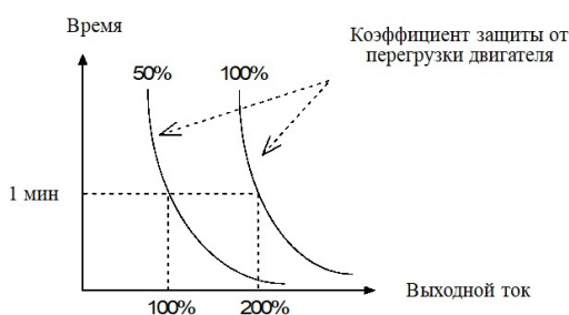
Рис. 6-28 Кривая защиты двигателя от перегрузки
