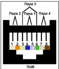
Рис. 3-19 Стандартный T568B
