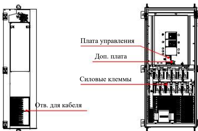
Рис.2-11 ITD...B3 (355~500 кВт)
