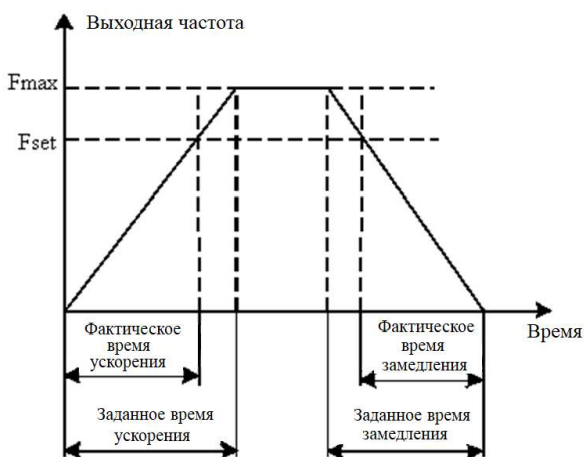
Рис. 6-2 Схема времени ускорения/замедления
