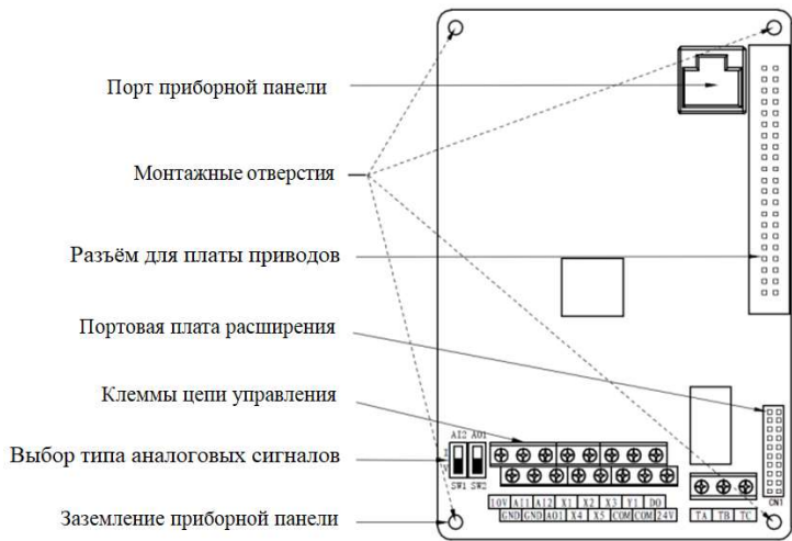
Рис. 3-16 Плата управления
