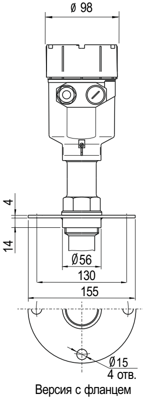
Версия с фланцем
