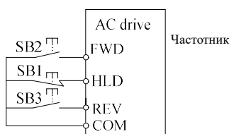
Рис.6-15 Трехпроводной режим управления 1
