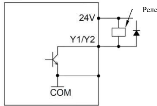
Рис. 3-16 Способ подключения внутреннего источника питания +24 В
