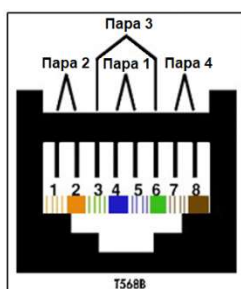
Рис. 3-19 Стандартный T568B
