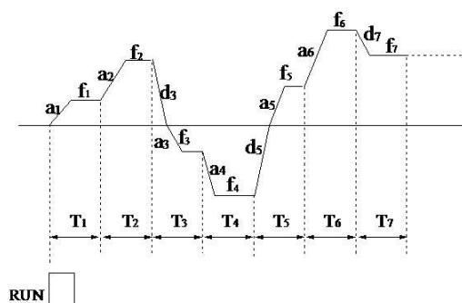
Рис. 6-26 Работа простого ПЛК
