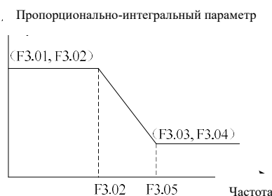
Рис. 6-7 Схема пропорционально-интегральных параметров контура скорости
