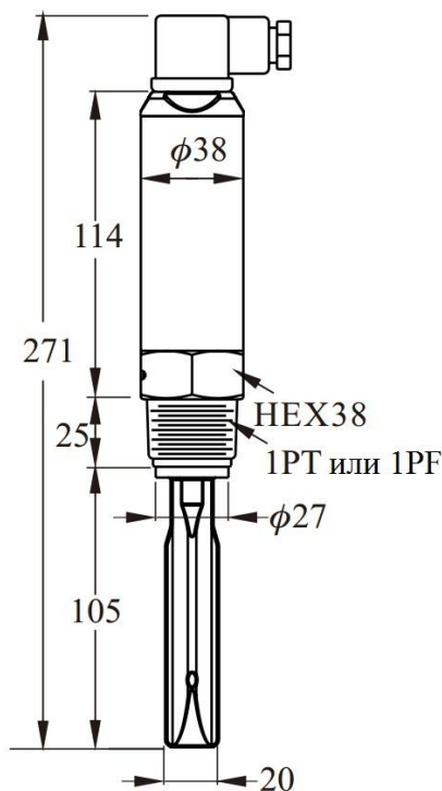
Рис.1 Размеры и тип электрического подключения
