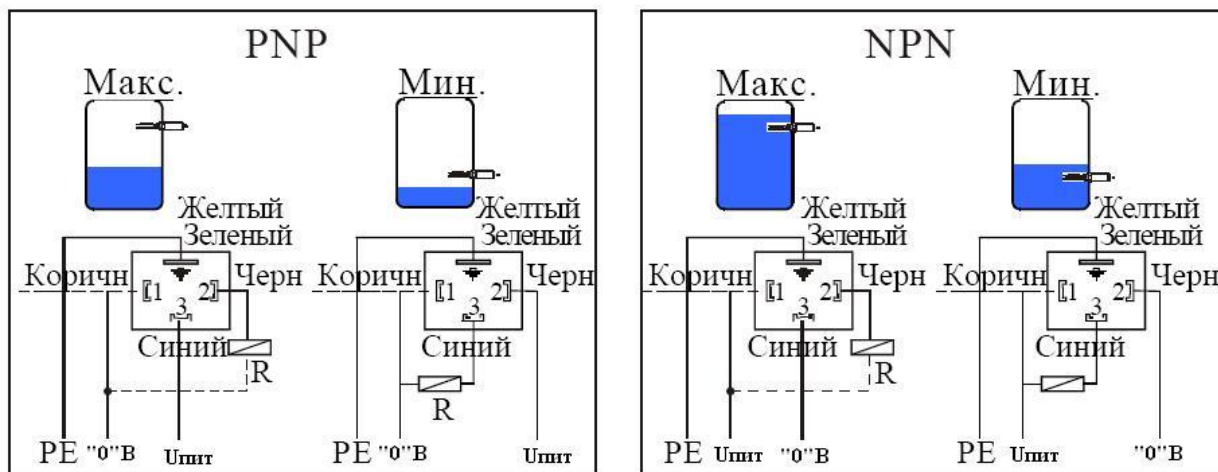
Рис. 2 Схема подключения
