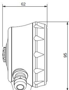
Вид сбоку, версия со штуцером снизу
